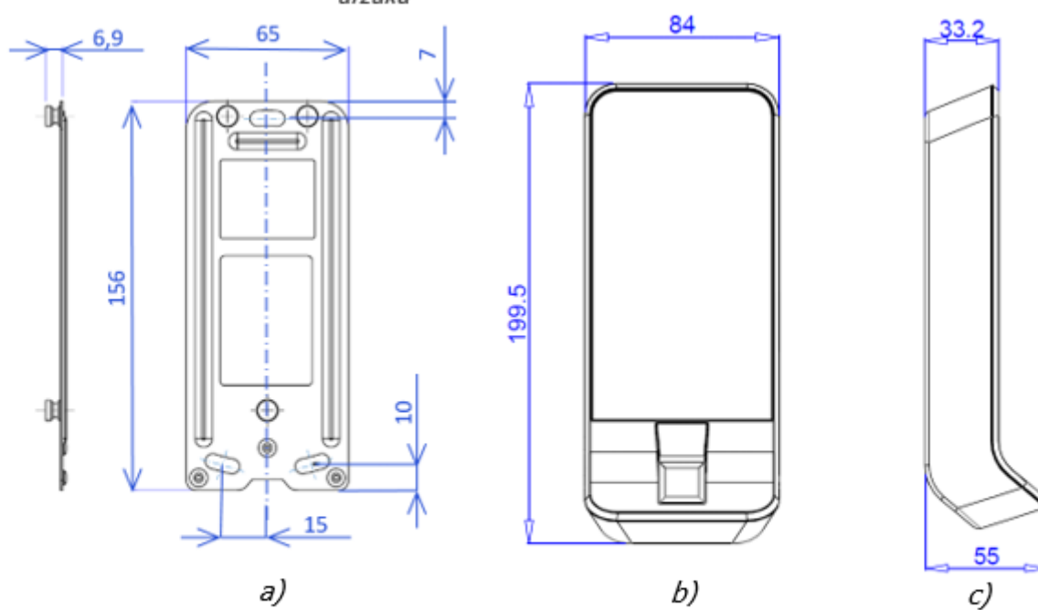
Obr. 3: Rozměry
