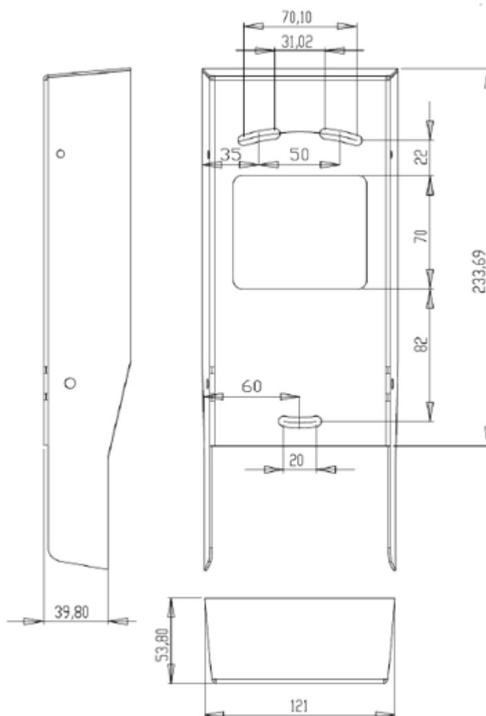
Obr. 5: Rozměry šasi
