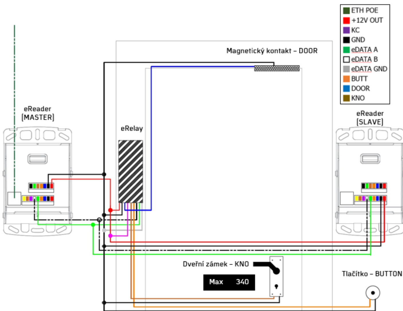
Obr. 395: Zapojení systému – varianta 4
